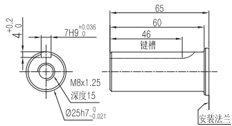
键槽轴 (公制)
