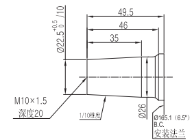
锥形轴 (公制)
