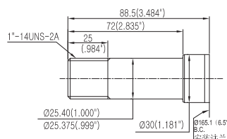
螺纹轴 (英制)
