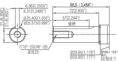
键槽轴 (英制)
