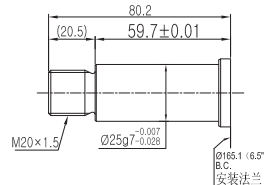
螺纹轴 (公制)
