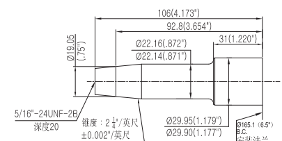
锥形轴 (英制)
