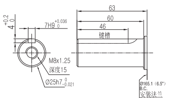
键槽轴 (公制)
