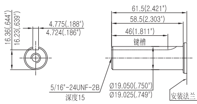
键槽轴 (英制)
