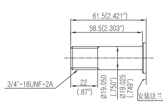
螺纹轴 (英制)
