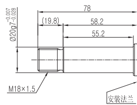
螺纹轴 (公制)
