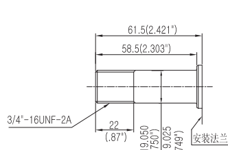
螺纹轴 (英制)
