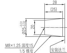
锥形轴 (公制)
