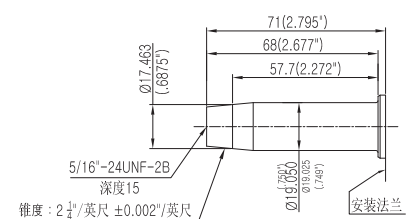
锥形轴 (英制)
