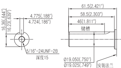
键槽轴 (英制)
