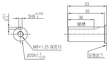
键槽轴 (公制)
