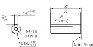
KEYWAY (JIS)
