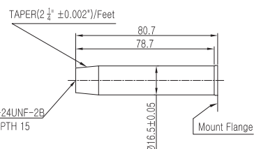
TAPER (SAE)
