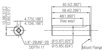
KEYWAY (SAE)
