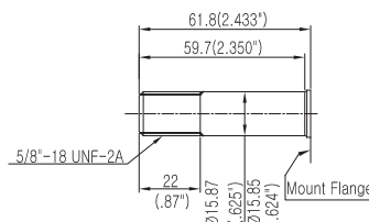
THREAD (SAE)
