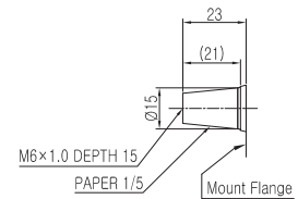
TAPER (JIS)
