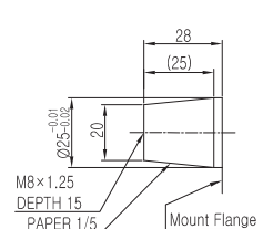
TAPER (JIS)
