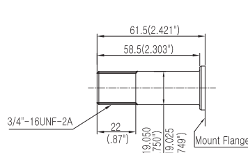
THREAD (SAE)
