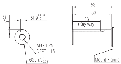
KEYWAY (JIS)
