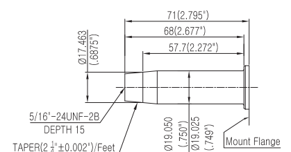
TAPER (SAE)
