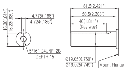
KEYWAY (SAE)
